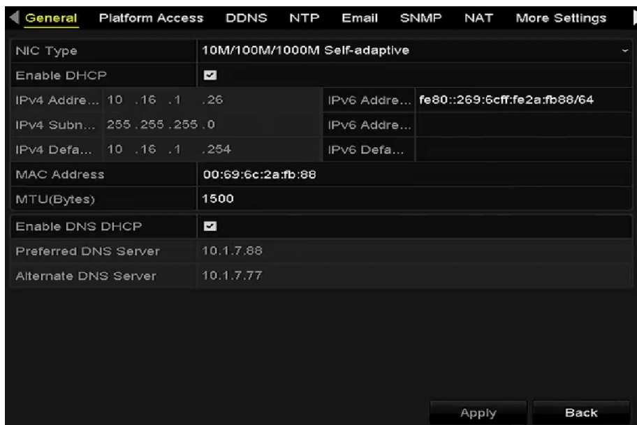
Рисунок 4.11 Сетевые параметры
