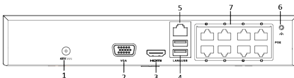
Рисунок 1.3 Задняя панель
