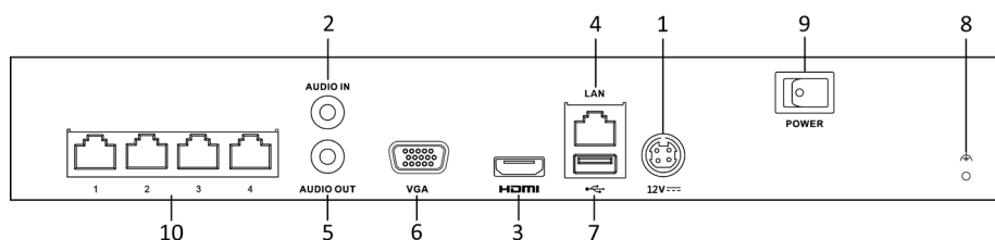
Рисунок 1.5 DS-N3XXP(B)
