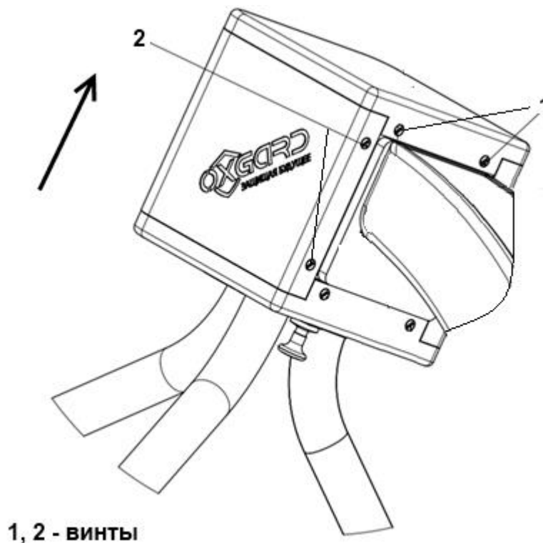
Рисунок 8 – Демонтаж защитного кожуха турникета
