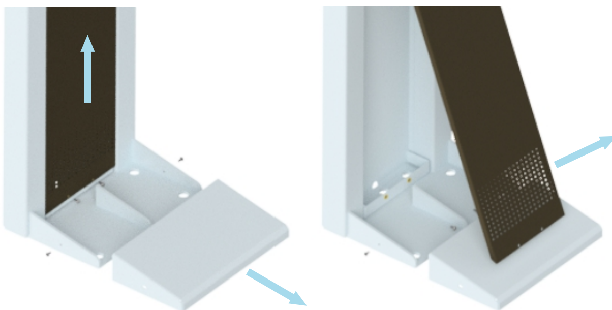
Рисунок 22 – Демонтаж центрального кожуха турникета
