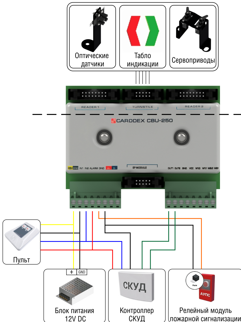
Рисунок 16 – Схема основных подключений турникета
