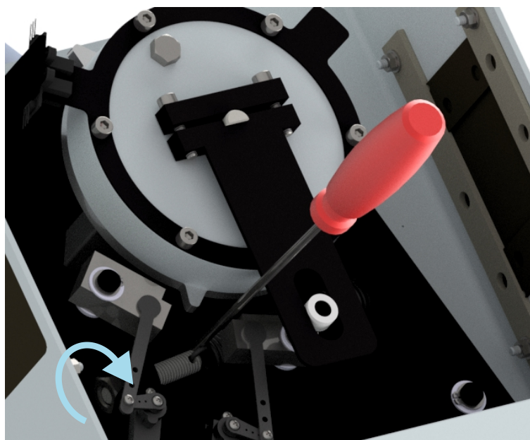
Рисунок 27 – Регулировка натяжения пружин
