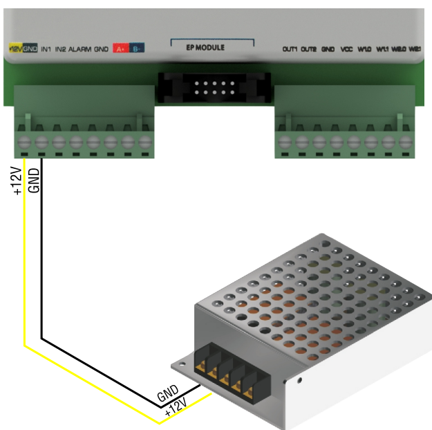
Рисунок 20 – Подключение питания к турникету
