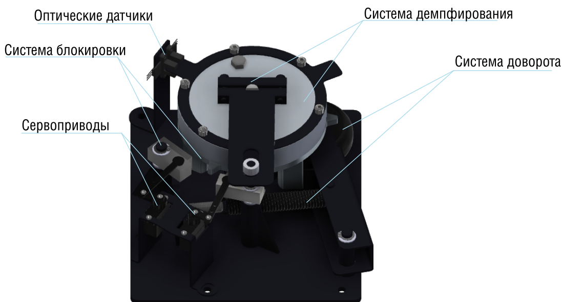
Рисунок 4 – Устройство механизма турникета
