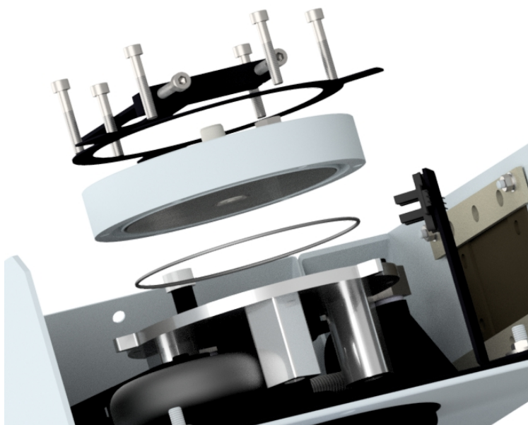
Рисунок 24 – Порядок замены уплотнительного кольца
