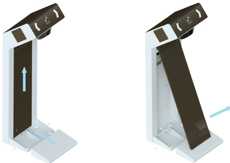
Рисунок 14 – Разборка кожухов турникета
