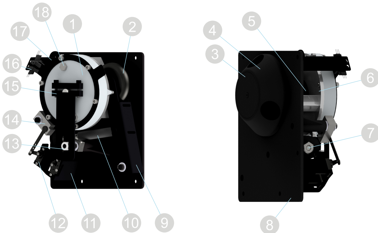
Рисунок 22 – Демонтаж центрального кожуха турникета
