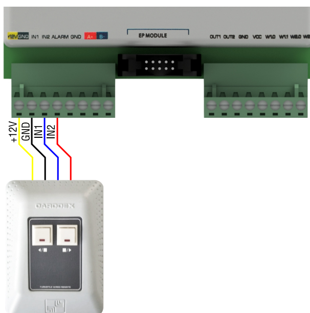
Рисунок 17 – Подключение ПДУ к турникету
