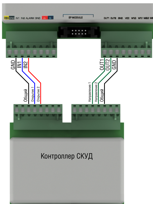
Рисунок 18 – Подключение турникета к стороннему СКУД
