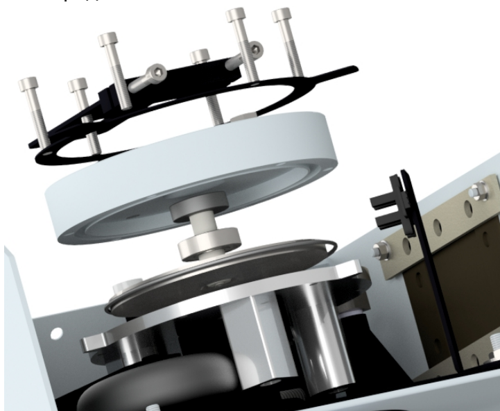
Рисунок 25 – Порядок замены сальника
