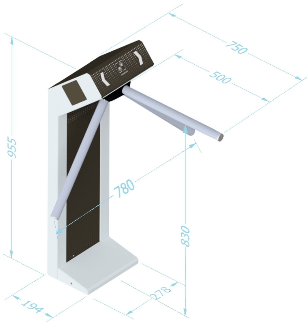
Рисунок 1 – Габаритные размеры турникета с планками
