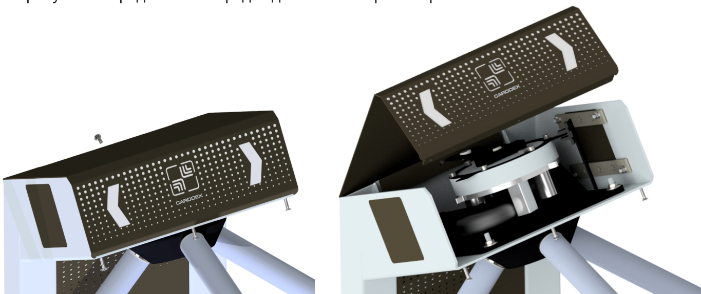
Рисунок 21 – Демонтаж верхней крышки турникета
