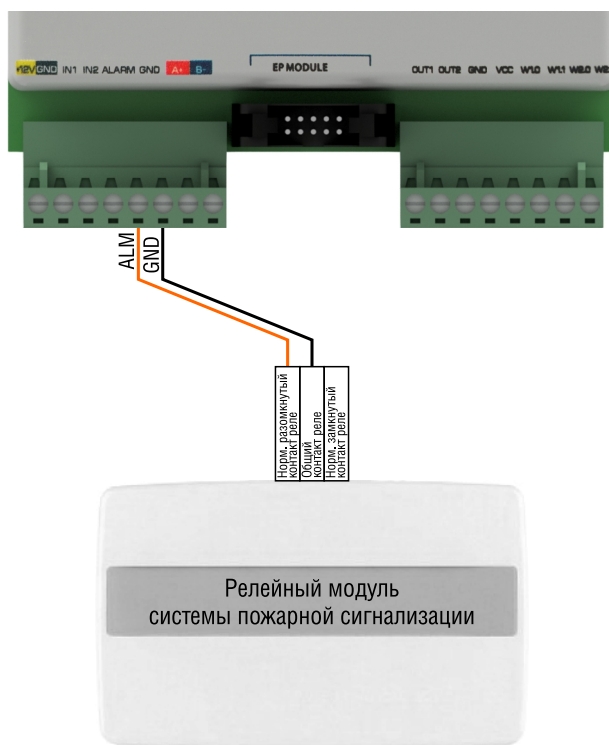
Рисунок 19 – Подключение АУПС к турникету
