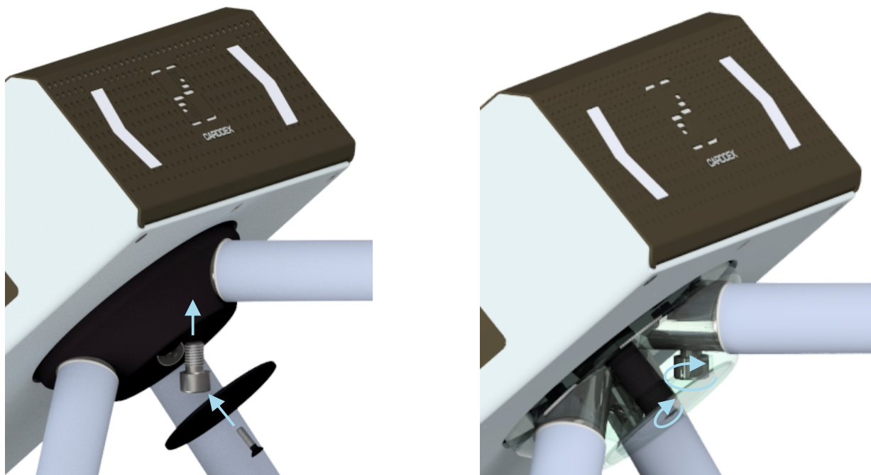
Рисунок 15 – Установка стандартной преграждающей планки
