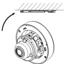
Рисунок 2-3 Установка камеры на потолок
