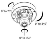
Рисунок 2-4 3-х осевая установка
