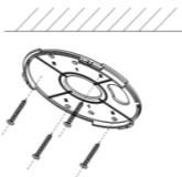
Рисунок 2-2 Крепление монтажной платформы
