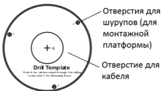
Рисунок 2-14 Шаблон крепления
