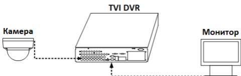
Рисунок 3-1 Схема подключения
