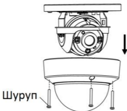
Рисунок 2-13 Разбор камеры
